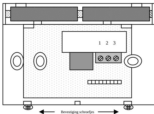
Tekening 1: Muur/Bodemplaat
